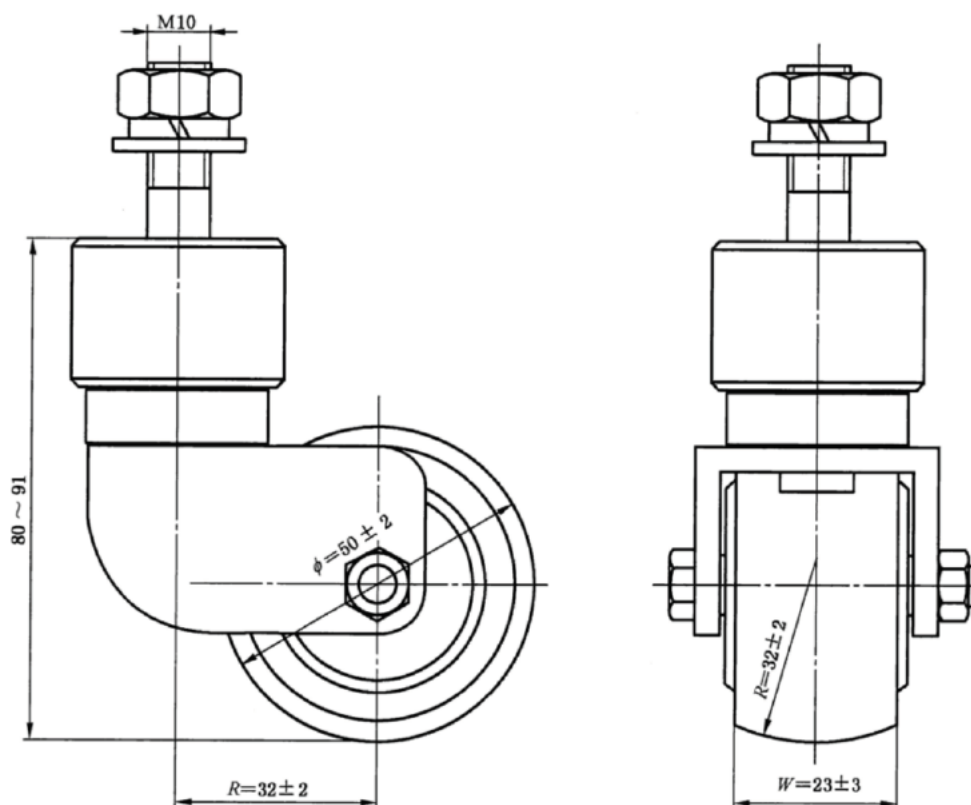
图 B.2 脚轮
