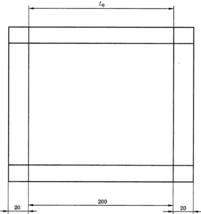
图 1 加热尺寸变化率画线示意图
